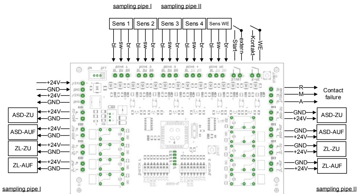
Fig. 3 Mainboard BMB 2000
